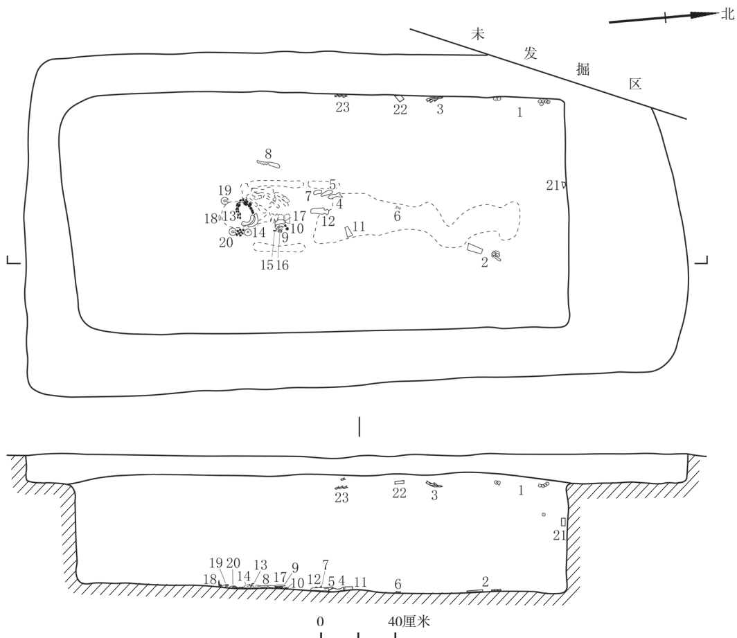
图二 M9平、剖图
