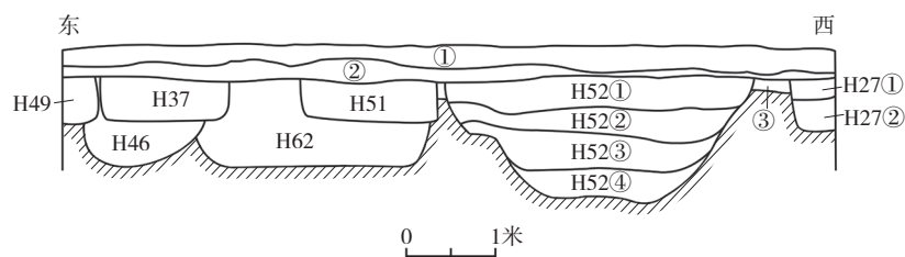
图五 T5042南壁剖面图
