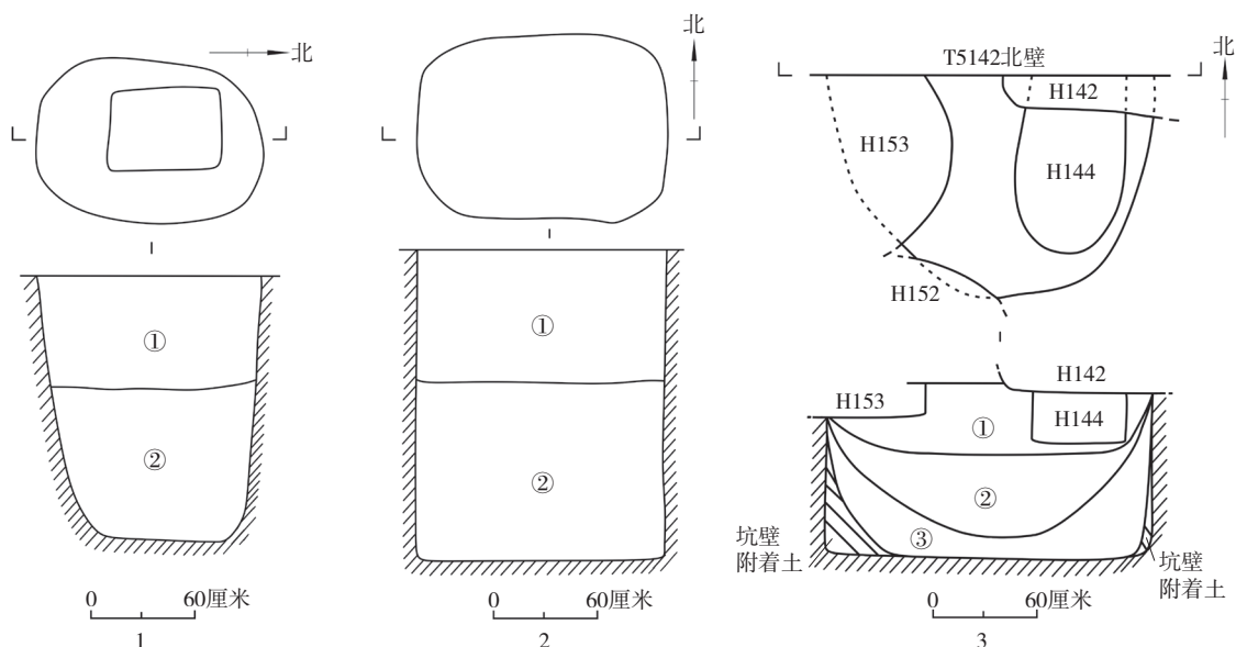
图一一 窖穴平、剖图 1. H75 2. H93 3. H194
