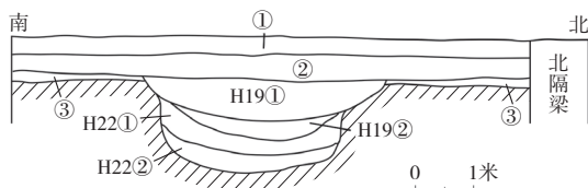
图三 T1413西壁剖面图
