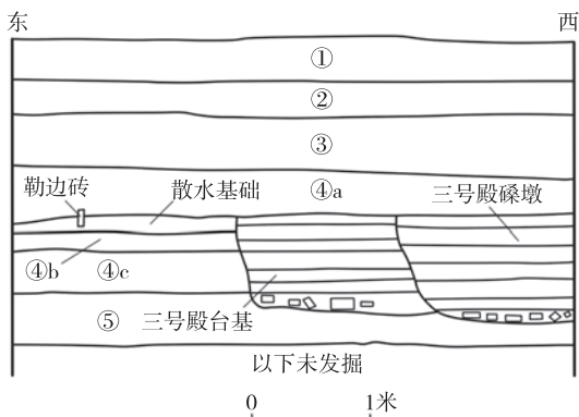
图二 TN02W17内TG1南壁剖面图
