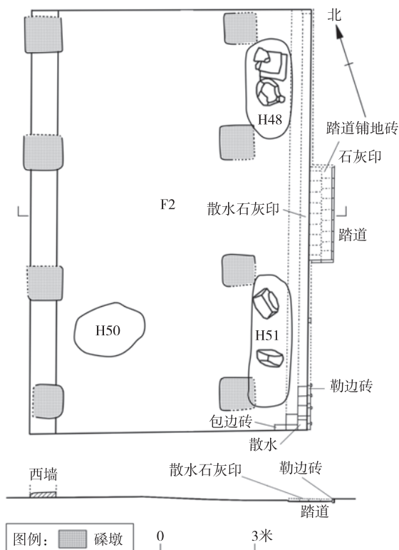
图六 F2平、剖面
