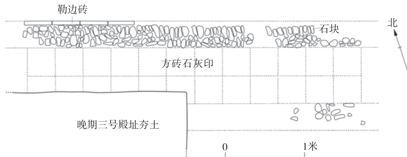
图八 砖石小路平面图
