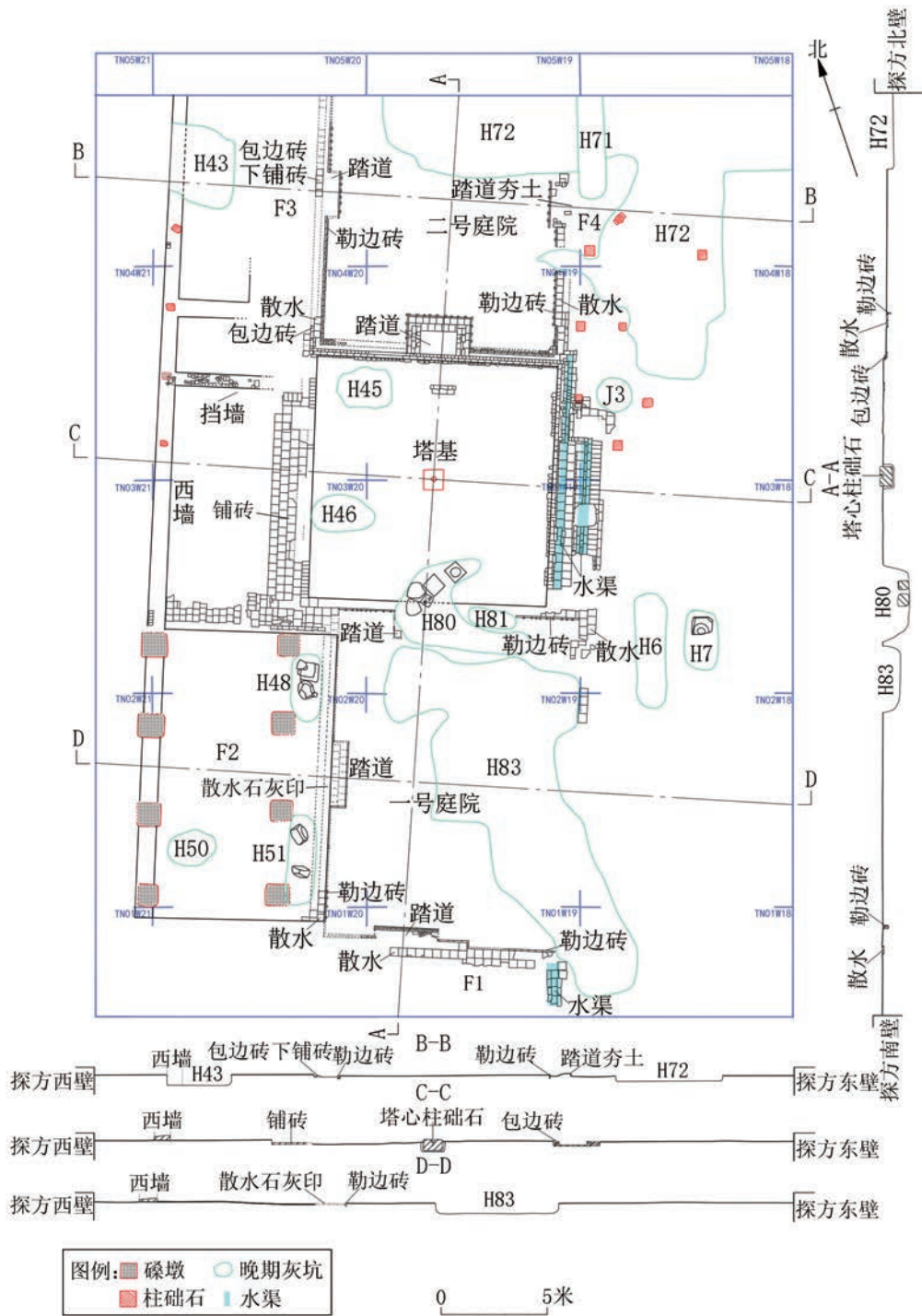
图三 晋阳古城唐代晚期后段建筑基址平、剖图
