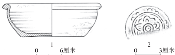
图一三 陶盆、盘
