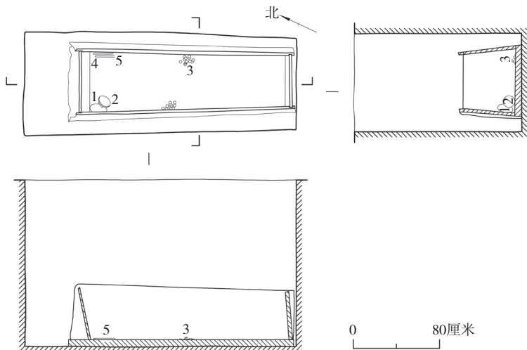
图一一 M68平、剖图 1、2.瓷碗 3.铜钱 4、5.铜发钗
