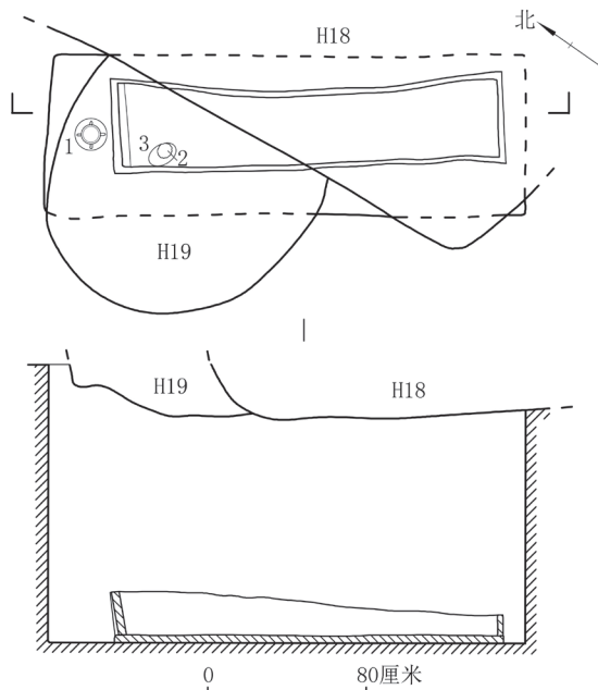
图七 M56平、剖图 1. 瓷四系罐 2. 瓷碟 3. 瓷碗
