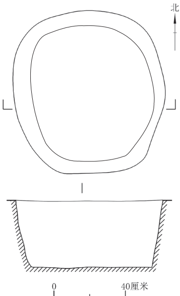
图三 H15平、剖面
