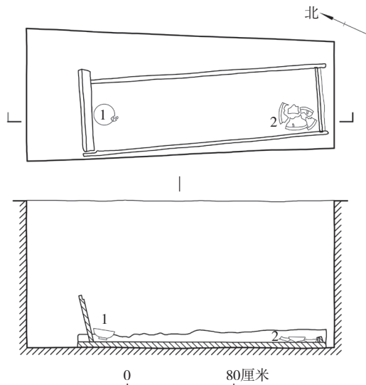
图一三 M70平、剖图 1. 瓷碗 2. 釉陶碗
