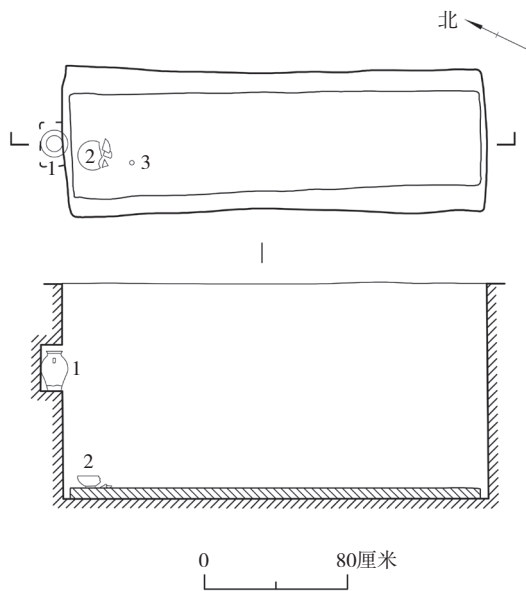
图九 M66平、剖图 1. 瓷四系罐 2. 瓷碗 3. 铜钱
