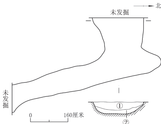
图六 G3平、剖面
