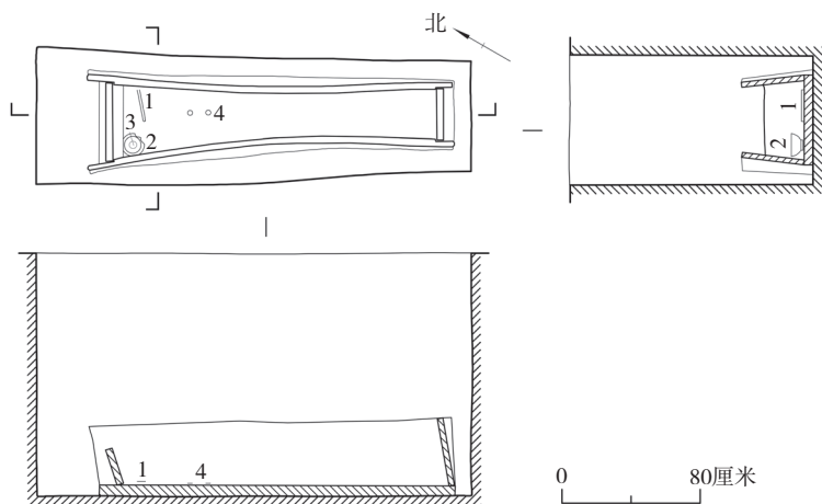
图一二 M69平、剖图 1. 铜发钗 2、3. 瓷碗 4. 铜钱
