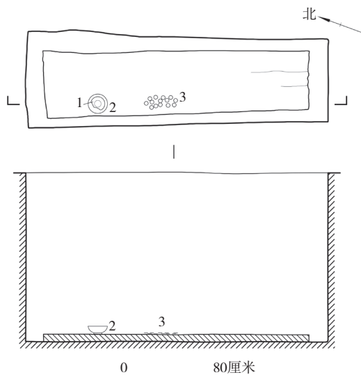
图一〇 M67平、剖图 1、2.瓷碗 3.铜钱
