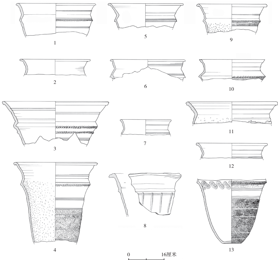
图一五 陶大口尊
