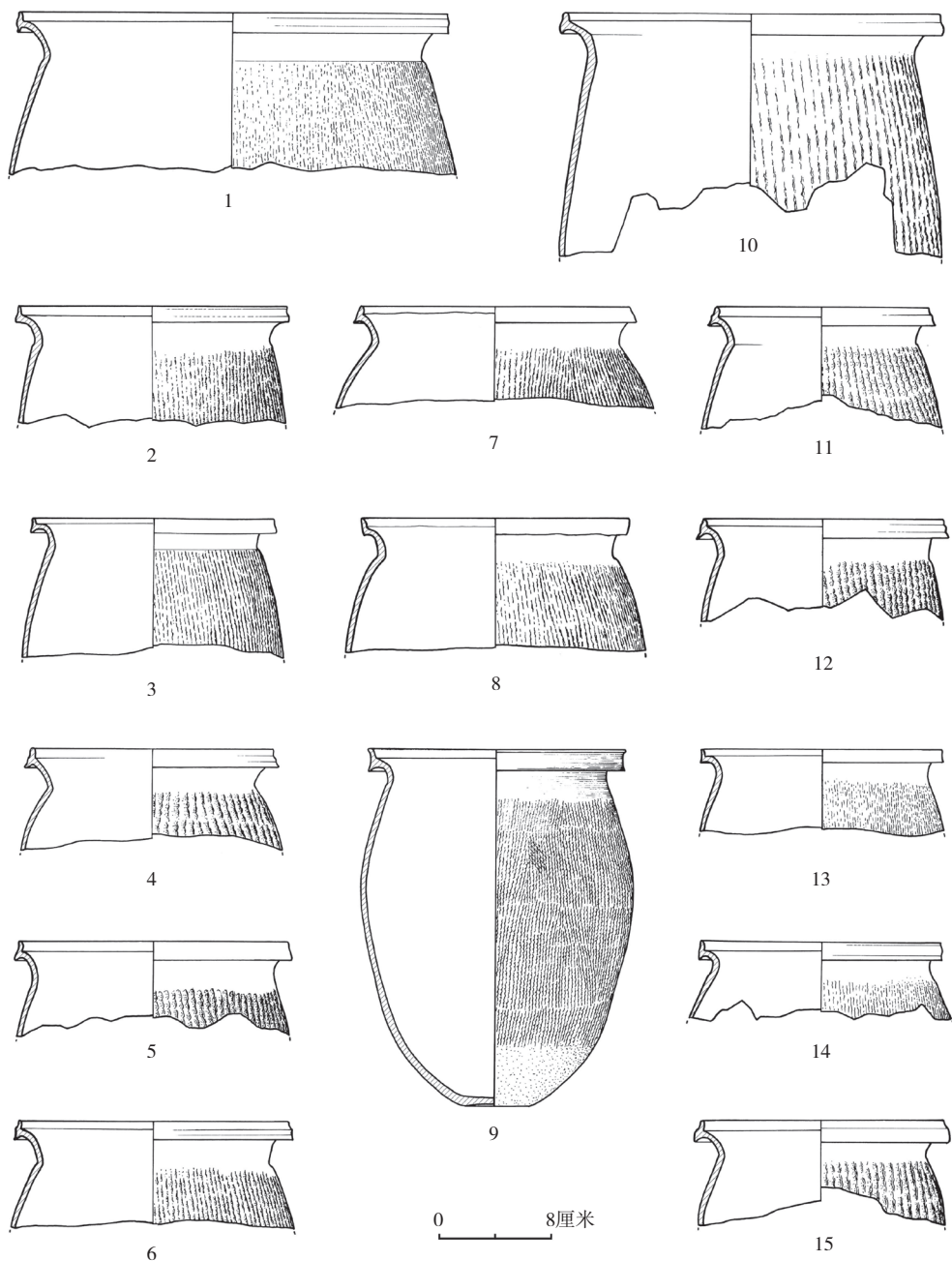
图一二 陶夹砂罐
